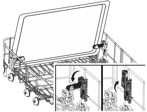
Abbildung 6: Backblech-Waschhalter
