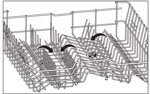
Abbildung 8: Klappbare Drähte im oberen Korb
